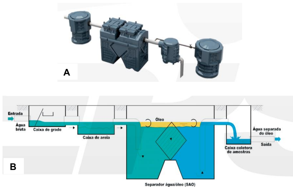
Figura 8 – (A) Sistema separador de água e óleo (SSAO). (B) Esquema genérico de funcionamento de um SSAO.
