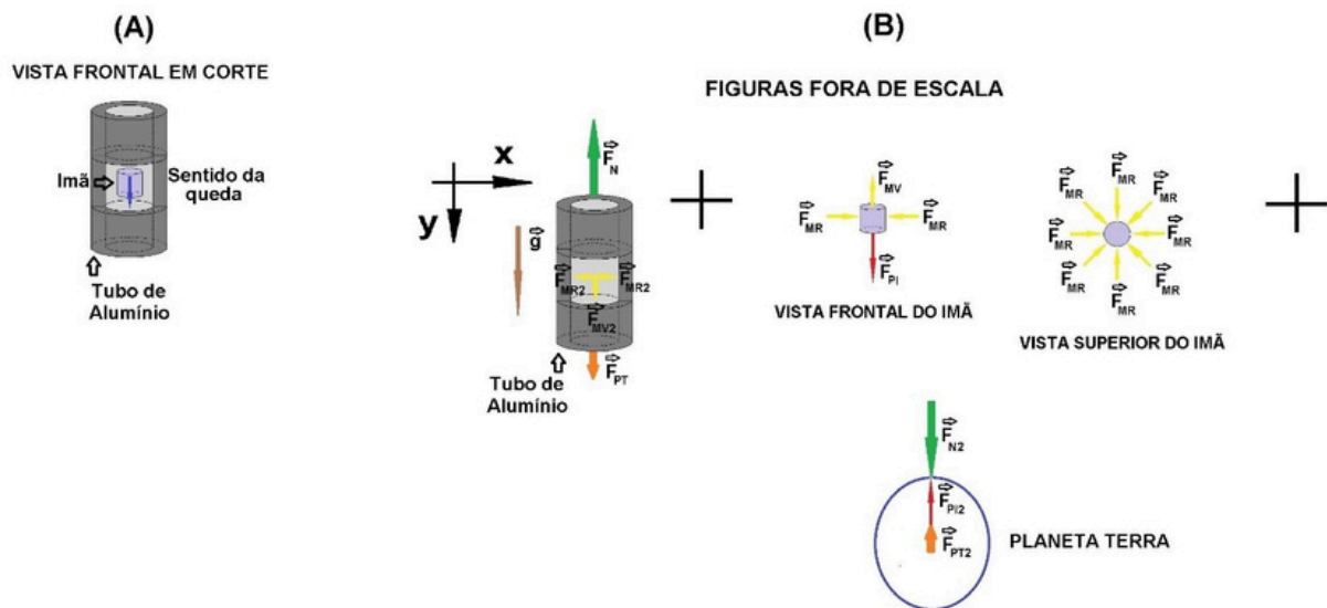
Figura 64 – Diagrama de Forças do ímã cilíndrico.
